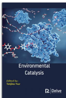
《环境催化》
