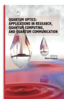
《量子光学》
