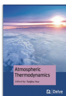
《大气热力学》
