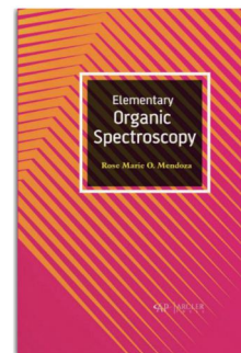
《有机光谱学》
