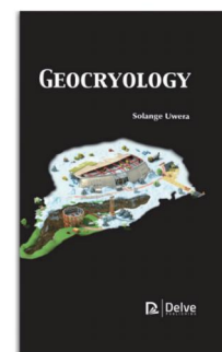
《地质学》
