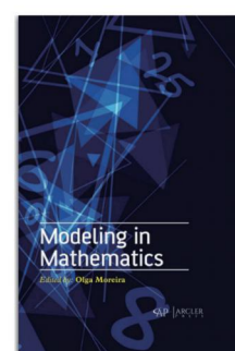
《数学建模》
