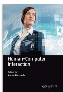
《人机交互》
